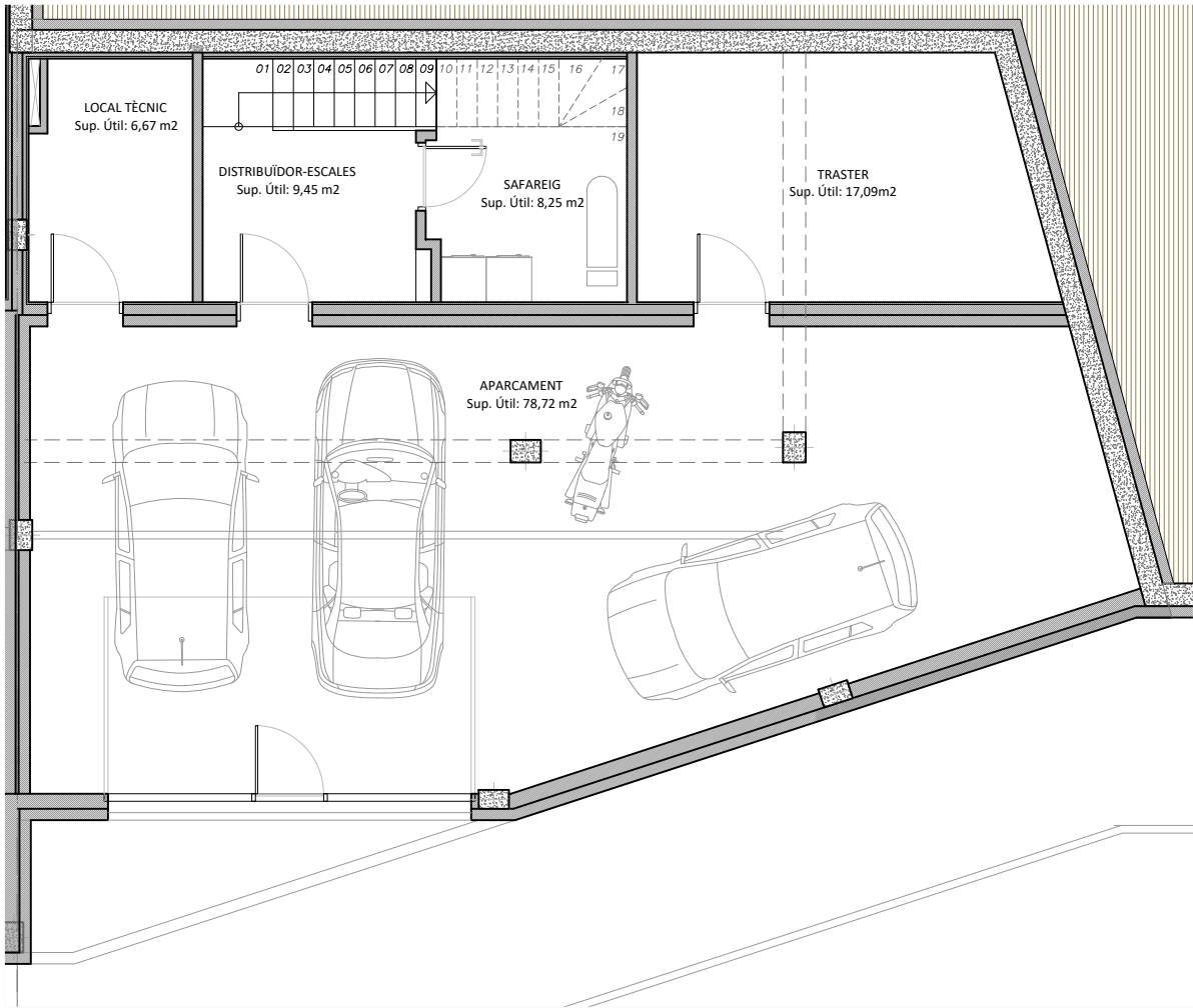
PLANTA SOTERRANI
