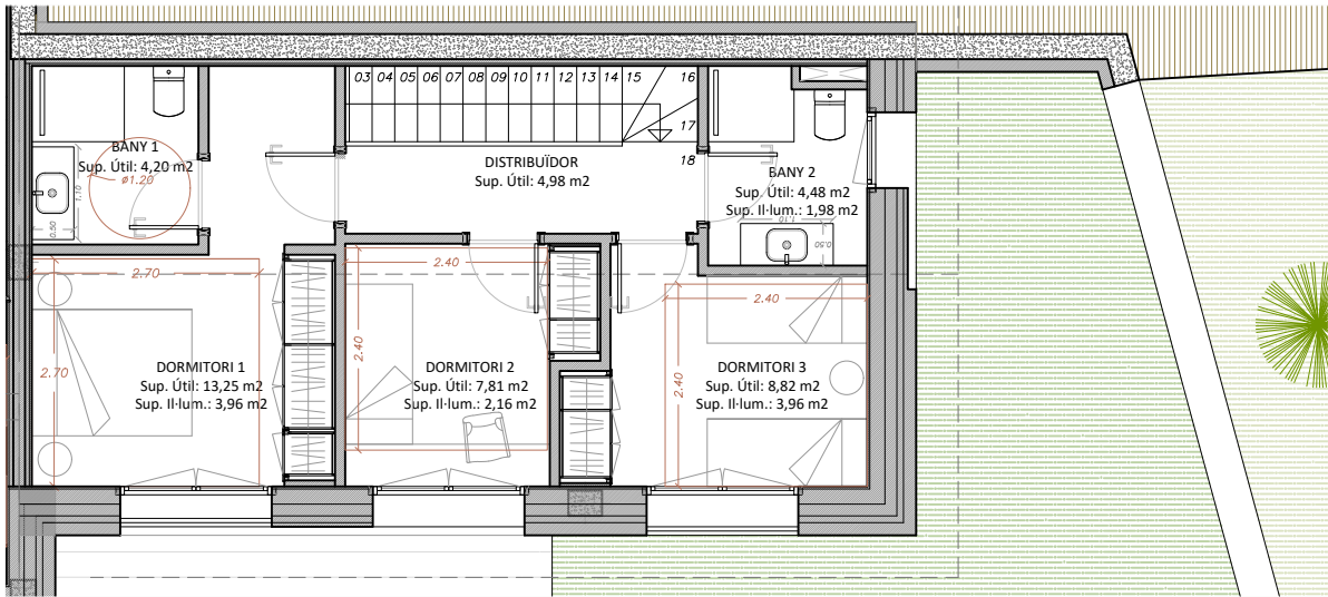
PLANTA PRIMERA
