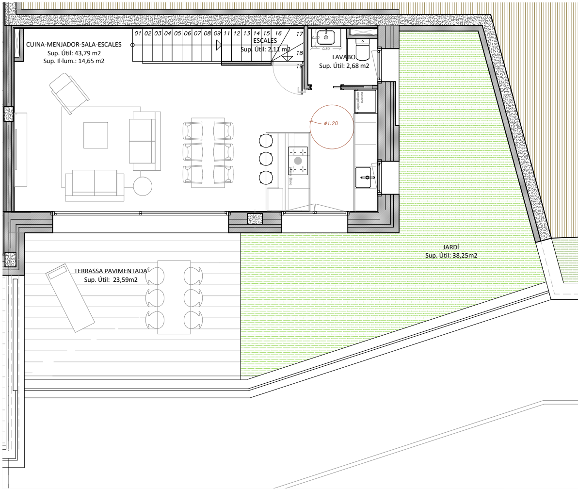
PLANTA BAIXA
